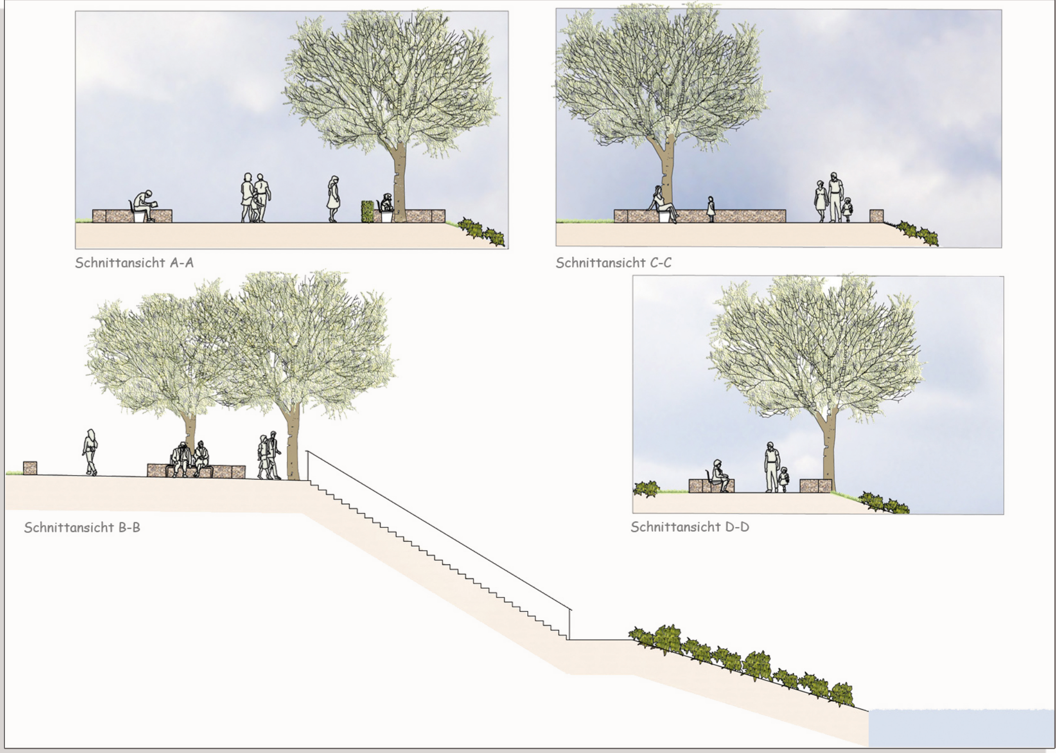
Schnittansicht
