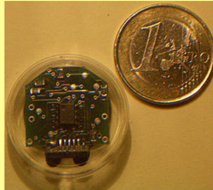
Elektronischer Temperaturschreiber
