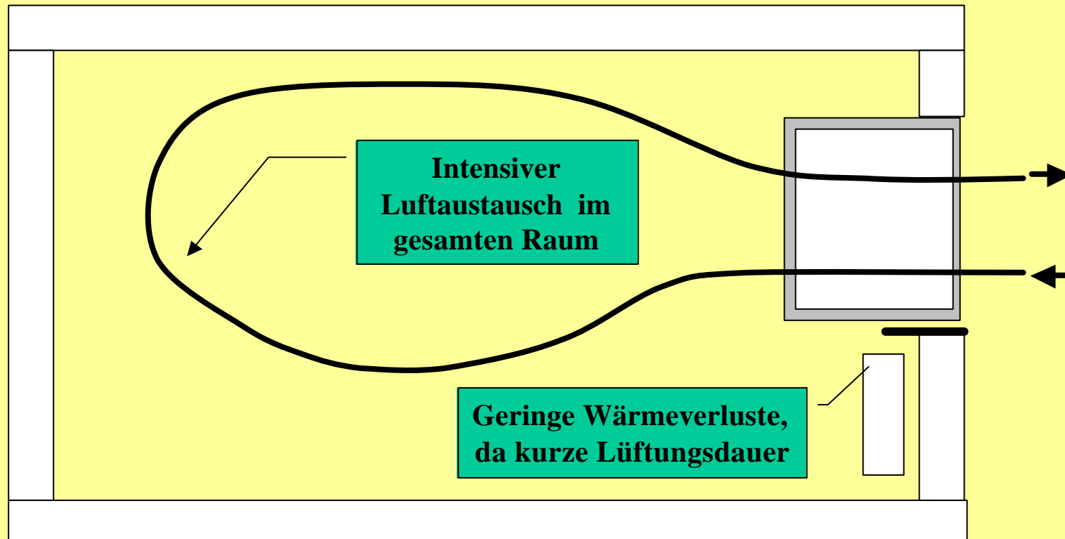
Klassenraum im Querschnitt (Raumtiefe 5-6 m)
